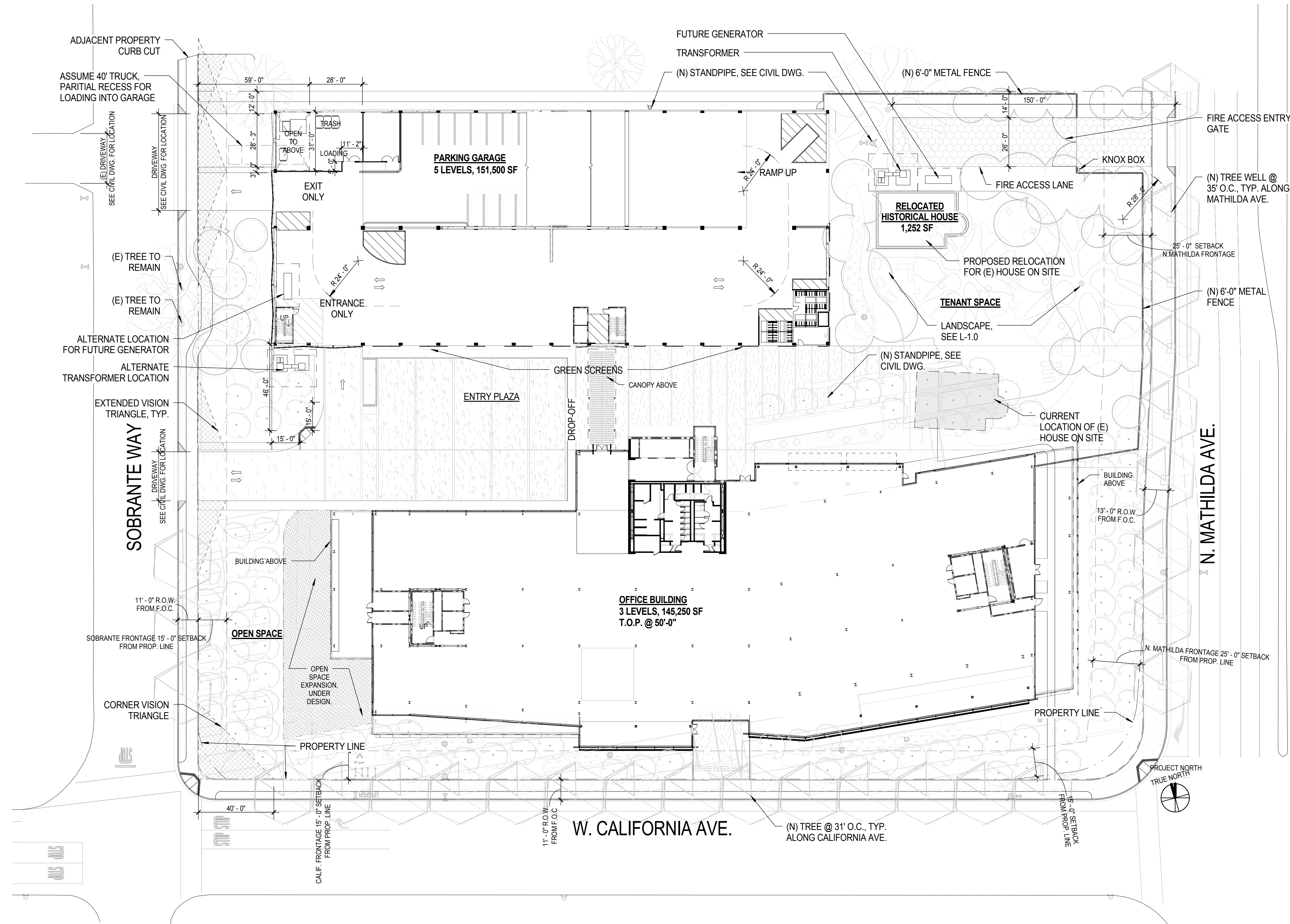
1 SITE PLAN (PRC) SCALE: 1" = 30'-0"
